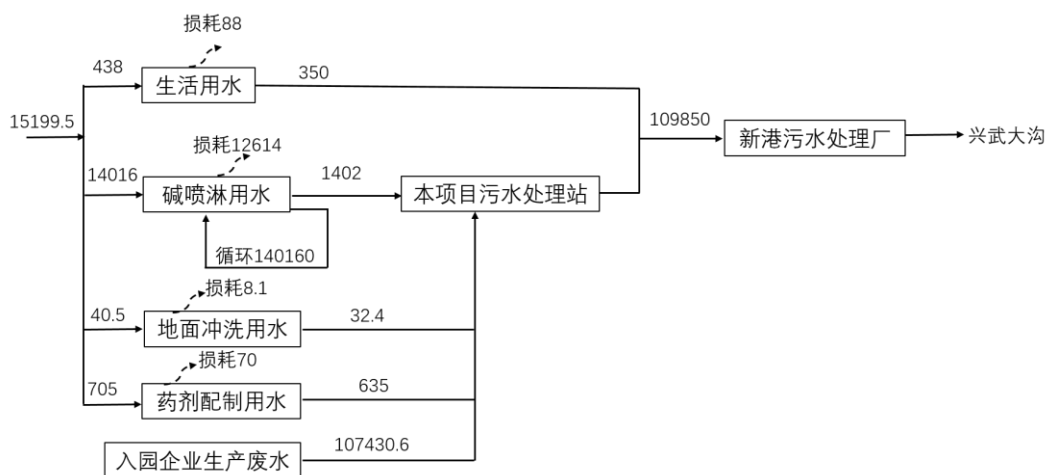
图 3.3-1 本项目水平衡（单位：t/a）
